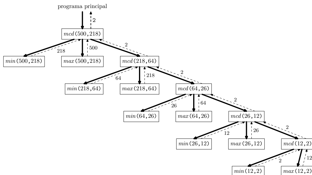
Figura 6.4: Árbol de llamadas para mcd(500, 218) .
