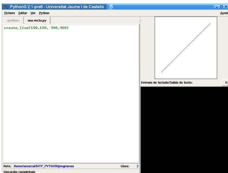
Figura 3.5: Programa que dibuja una recta en la ventana gráfica del entorno PythonG.
