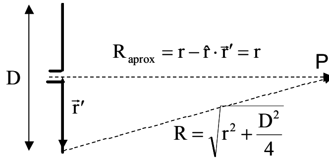
Figura 1.9: Error de fase de una antena
