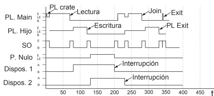
Figura 1.8 Caso de procesos ligeros
