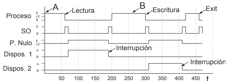
Figura 1.6 Caso de un solo proceso
