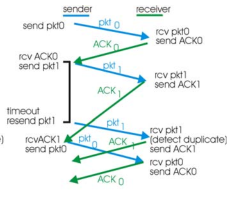
(d) premature timeout
