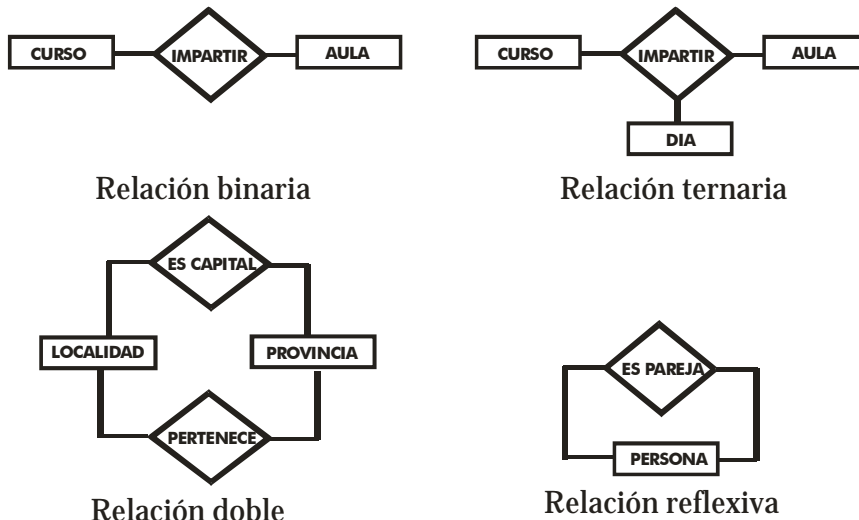
Ilustración 16, Tipos de relaciones
