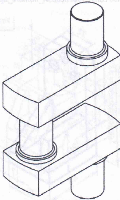
Figura 8.4. Representación de un cigüeñal.
