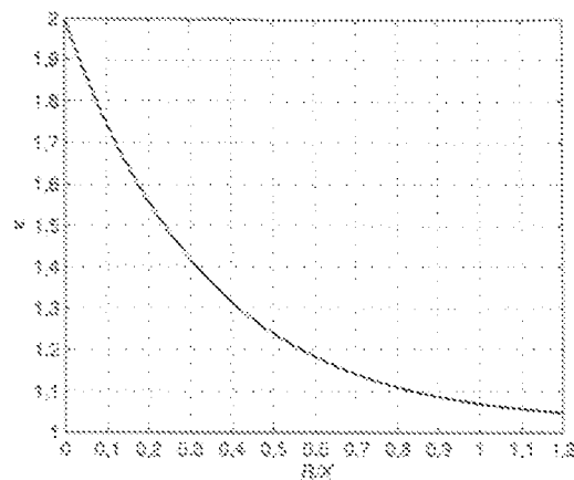
Figura 4.A. Parámetro \kappa para el cálculo de la corriente de corto según la norma UNE-EN 50306.
